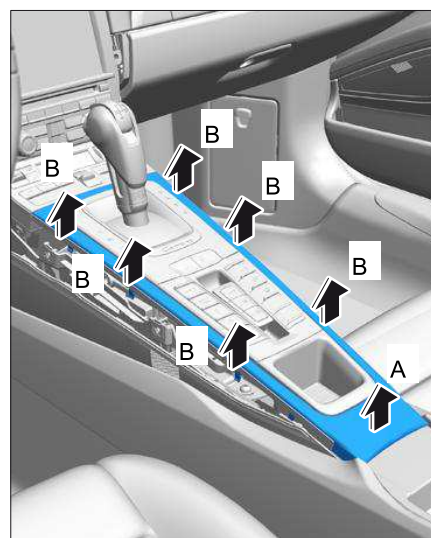
拆卸中控台盖
