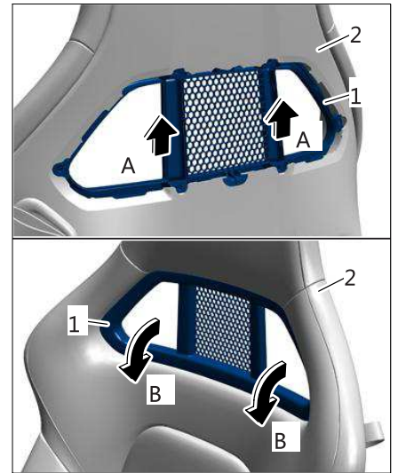
拆卸前饰板
