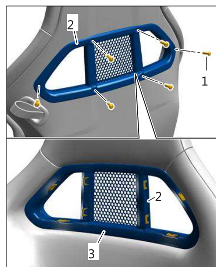
拆卸后饰板
