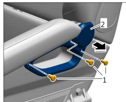
拆卸下部安全带导槽（以外侧下部安全带导槽为例）
