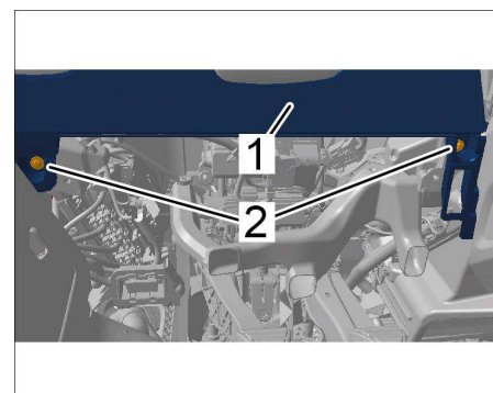
松开仪表板下面饰板的底部
