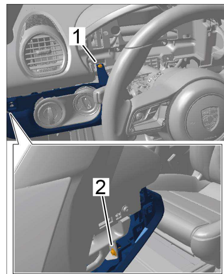
松开仪表板下面饰板的顶部
