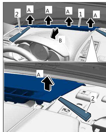
拆卸仪表板盖（除霜器装饰件）
