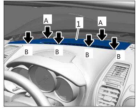
安装仪表板盖（除霜器装饰件）
