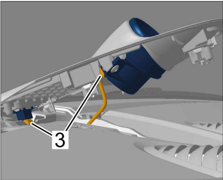
拆卸音箱饰板
