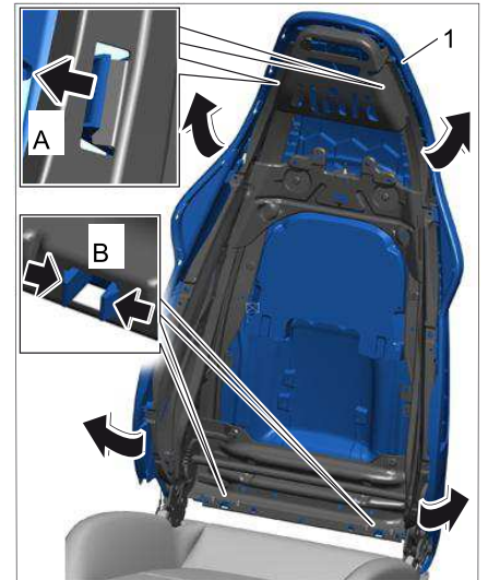
拆卸座垫托架
