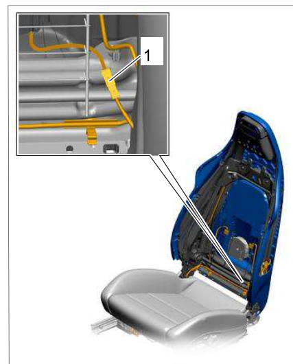
断开电气插头连接
