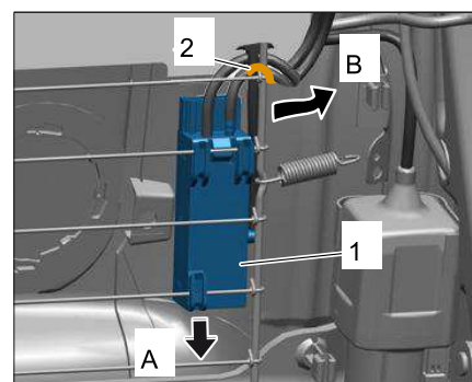
拆卸腰部支撑调整控制阀
