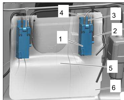
连接空气连接管路
