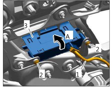
拆卸记忆座椅调节开关
