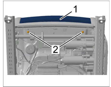
拆卸座椅加长件
