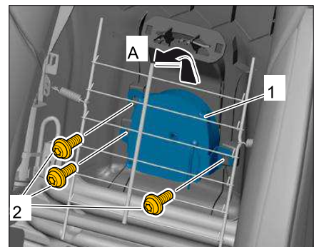
拆卸排风扇
