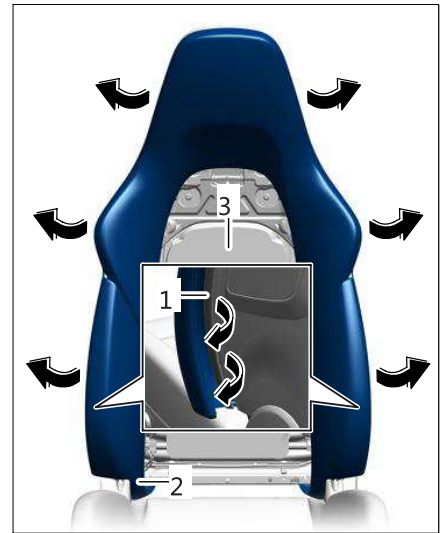
松开前排靠背衬垫
