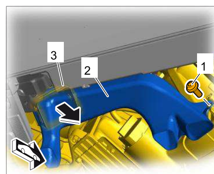
拆卸乘客侧前脚坑出风口
