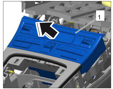
拆卸空调系统控制单元
