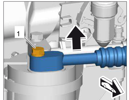
松开干燥器处的制冷剂管路
