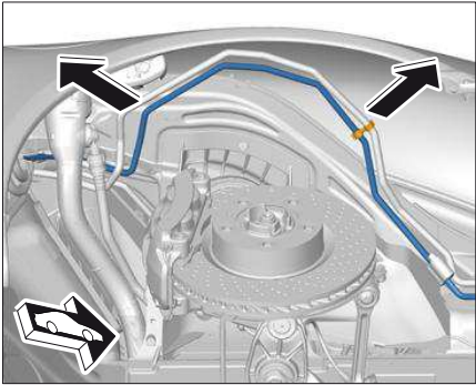
松开制冷剂管路
