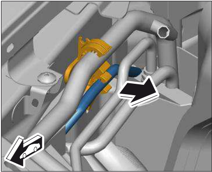
拆卸制冷剂管路
