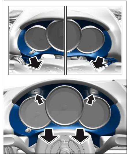
拆卸仪表板插入件
