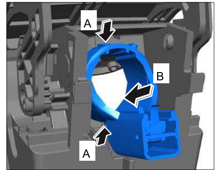
拆卸车灯单元
