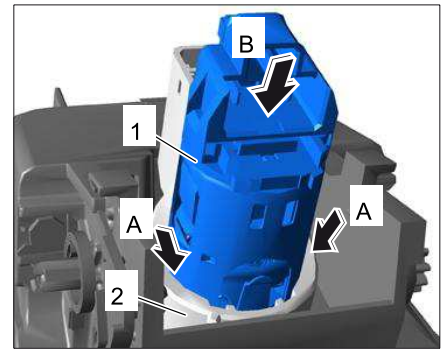
拆卸点烟器芯
