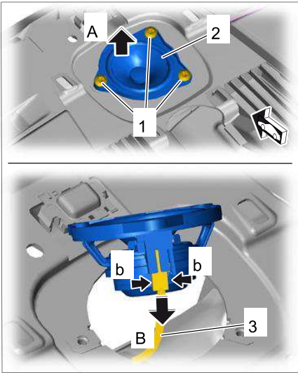
拆卸前中央音箱
