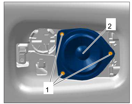
拆卸后音箱
