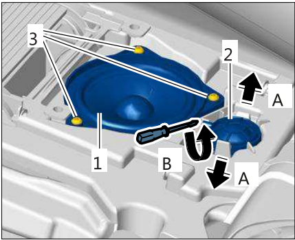
拆卸后音箱
