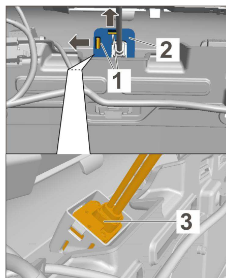
拆下倒车摄像头
