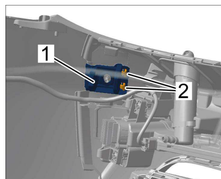
拆卸移动通信天线
