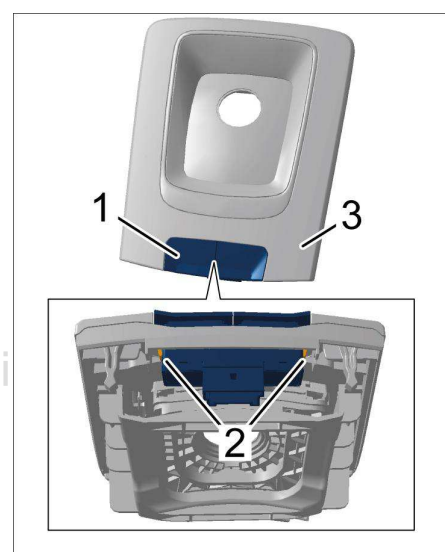
拆卸警示灯开关
