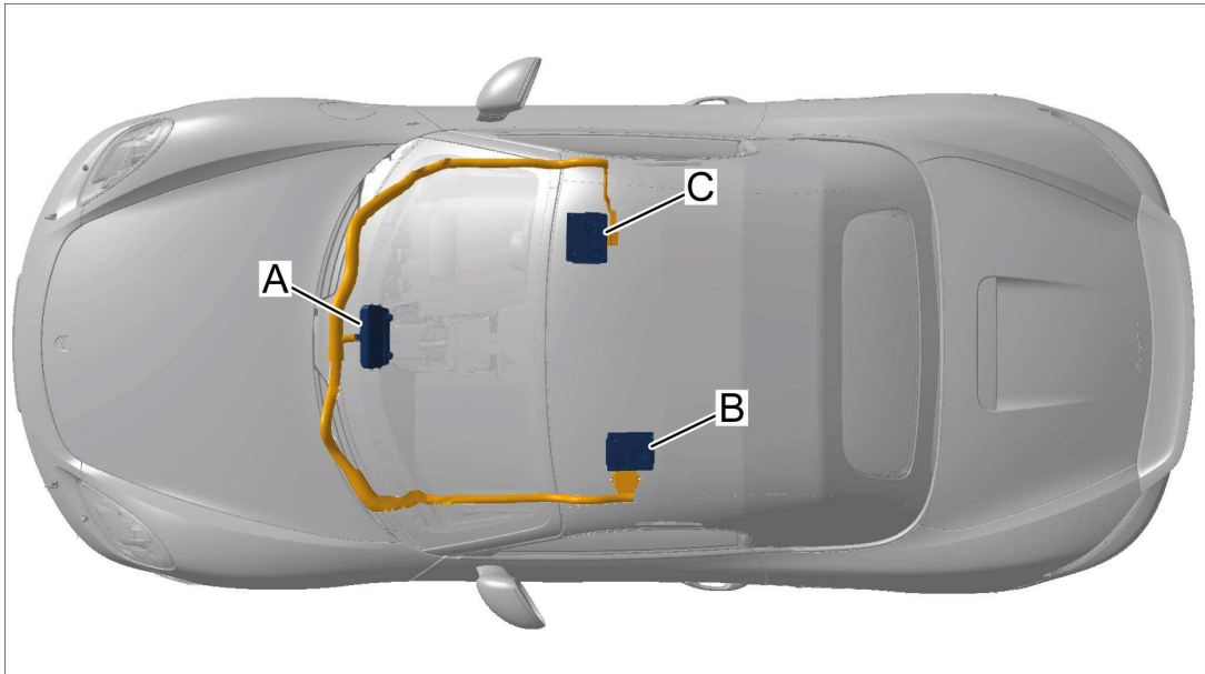
光纤（PCM 到音箱放大器和电视调谐器）的安装位置
