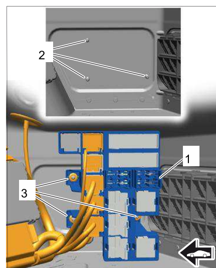
固定行李厢右侧的继电器座
