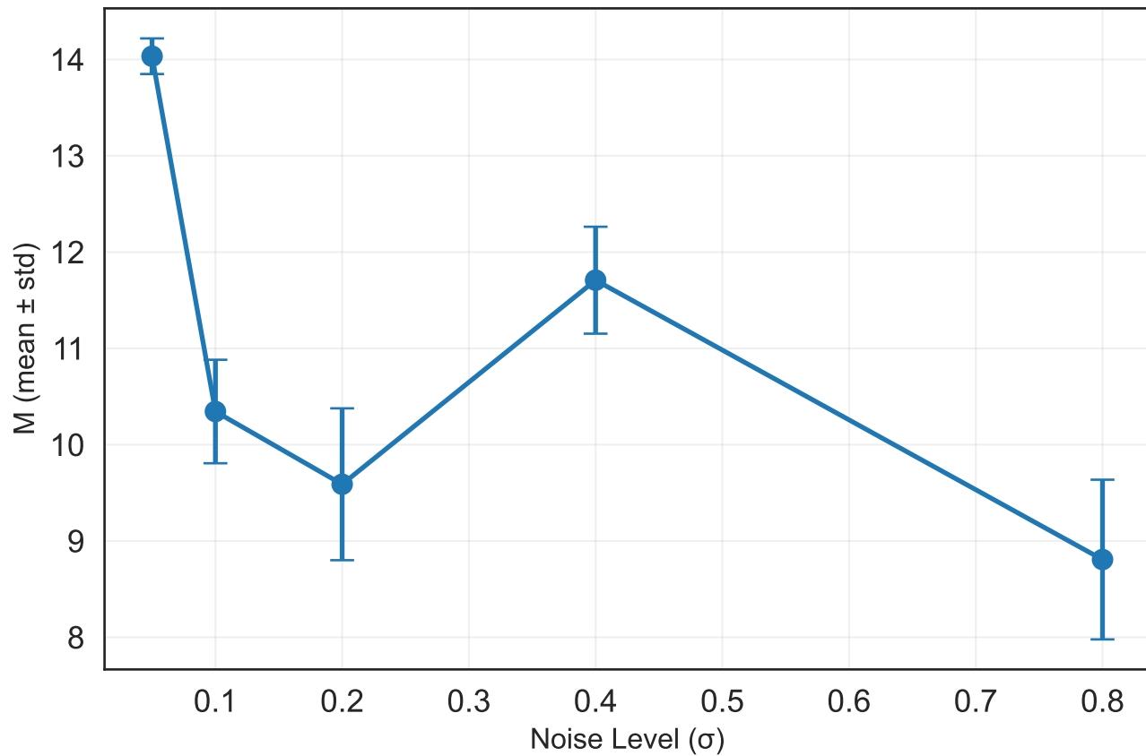
Occam's Razor: Posterior M vs Noise Level
