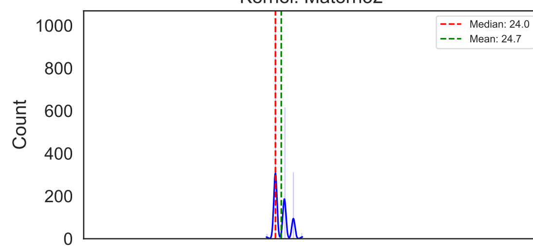
Kernel: Matern32
