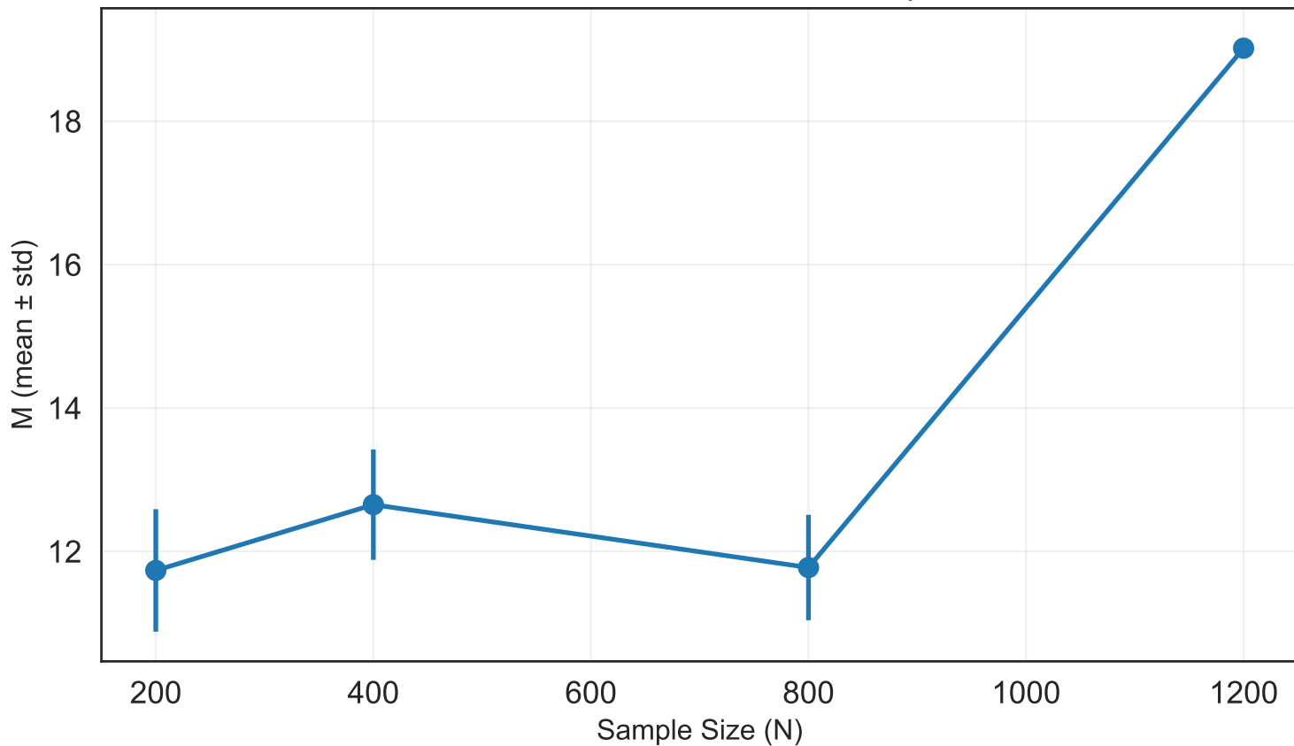
Occam's Razor: Posterior M vs Sample Size
