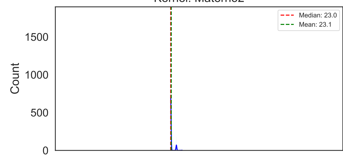
Kernel: Matern52
