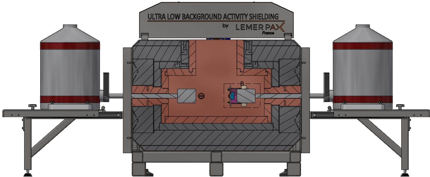
SECTION A-A SCALE 1 : 16
