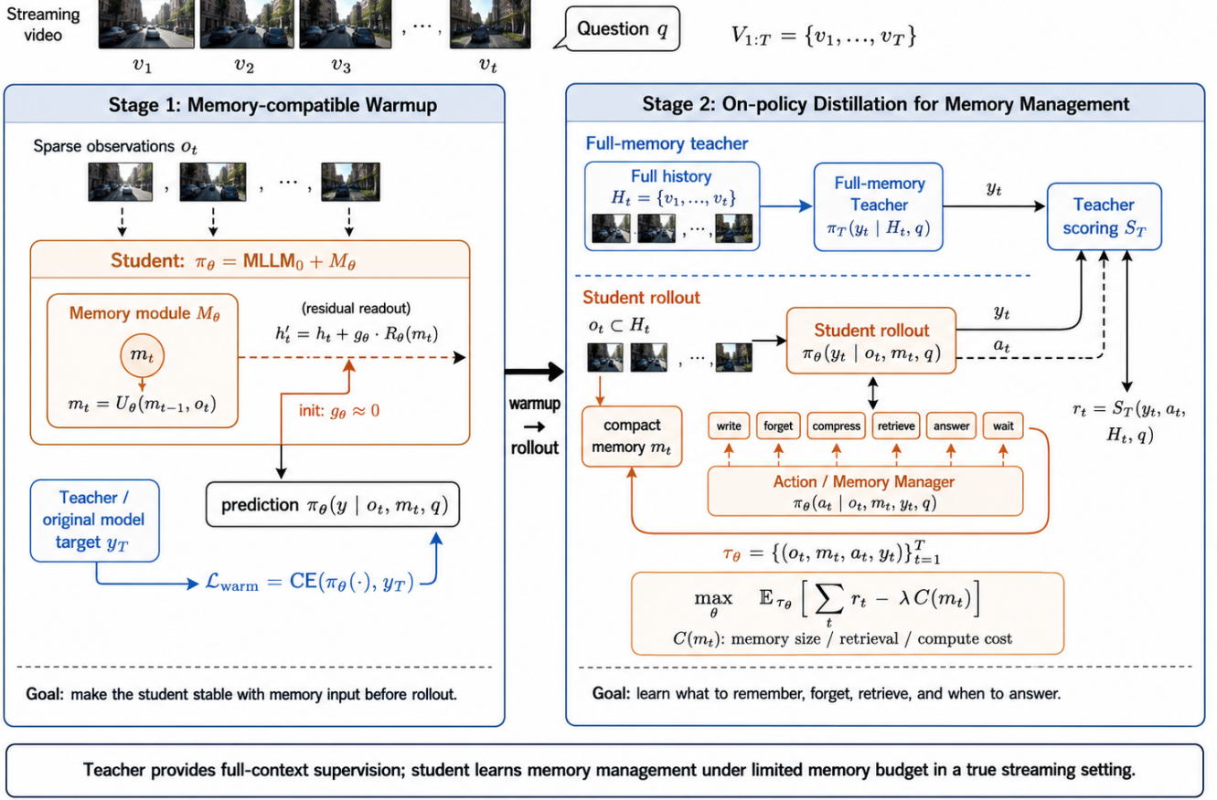
图 2: 可学习 Streaming Memory Manager 的初步方案。Teacher 不使用最近 32 帧, 而是在每个时刻从 t = 0 到当前 t 的完整因果前缀中均匀抽取 32 帧。这样视频变长后仍能覆盖早期、中段和当前内容, 为只保留 compact memory 的 Student 提供全局监督。该图为尚未实现的 proposal, 由 OpenAI GPT Image 2 辅助绘制, 不属于本文 Training-free 实验结果。
