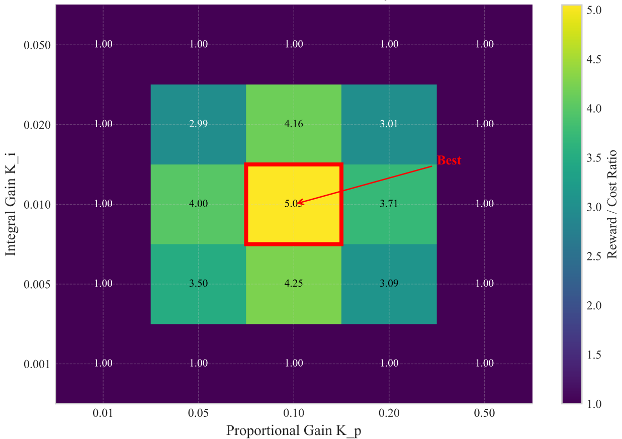
PID Parameter Ablation Study
