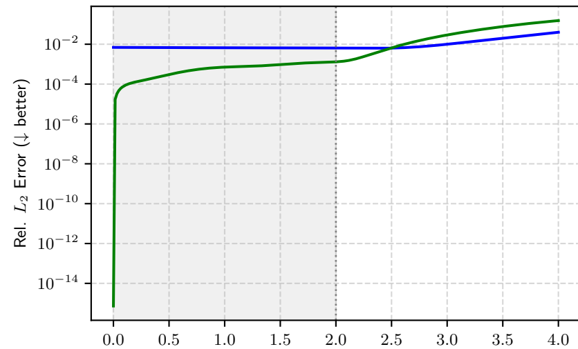
2D Poisson PDE
