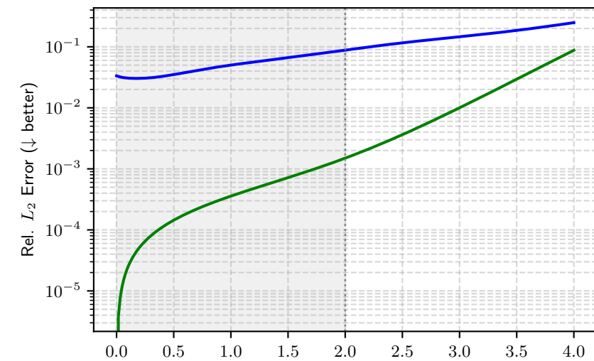
1D Fokker-Planck PDE
