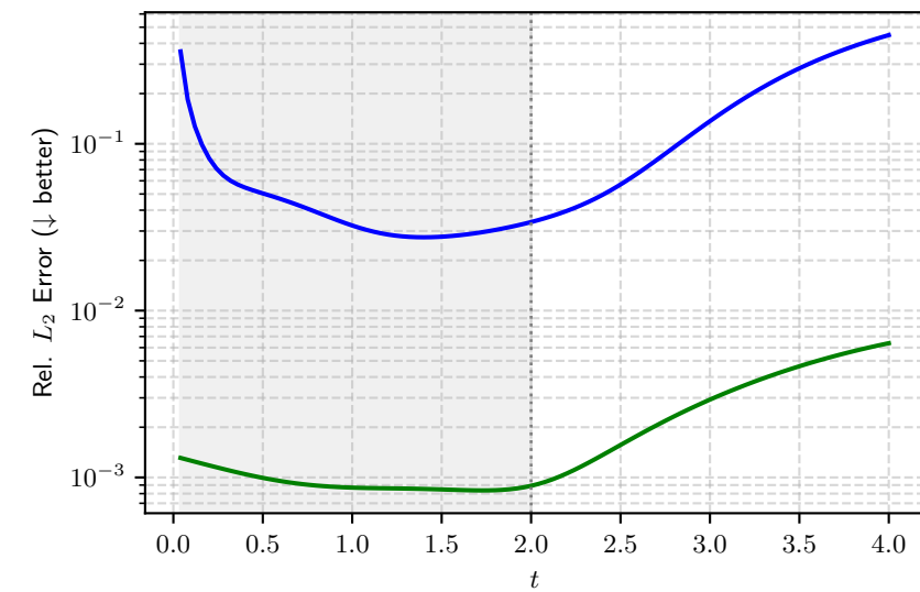
2D Poisson PDE
