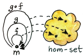
作为态射的么半群态射集和作为集合中的点。
