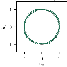
(d) 回拉单位圆 \kappa(\hat{A}) = 45.24
