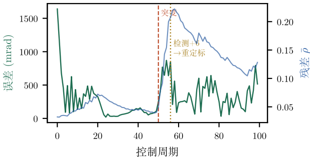
(b) 残差触发检测与恢复重定标
