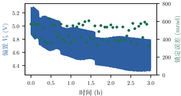
(a) 长期稳定性 3.0 h: 偏置跟踪 0.98 V 漂移, 重定标 0 次
