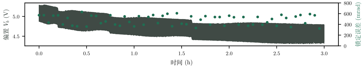
(a) 长期稳定性 (3.0 h, 偏置漂移 0.98 V, 重定标 0 次)
