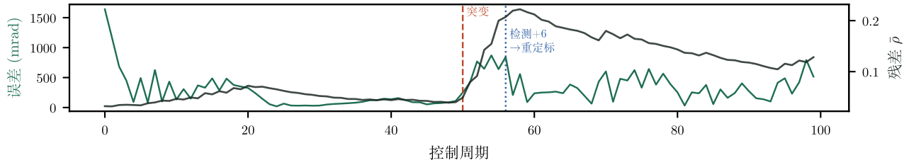
(b) 残差触发检测与恢复
