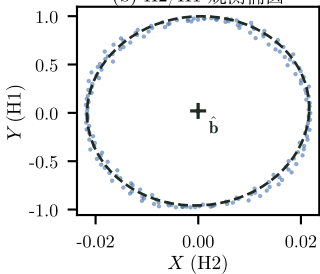
(b) H2/H1 观测椭圆
