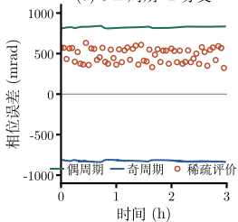
(a) 3 h 周期--2 分支
