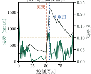
(b) 残差触发重扫
