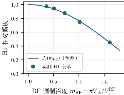
(a) 谐波随 RF 的 J_0 衰落 ( V_{\pi}^{\text{RF}} \approx 2.8 \text{ V} )
