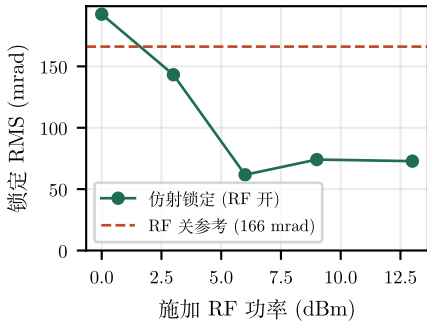
(b) 任意点锁定 RMS vs RF 功率
