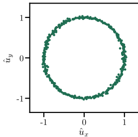
(b) 仿射回拉单位圆
