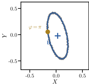
(a) 原始观测平面
