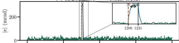
(a) 锁定误差 (第1200周期注入突变)
