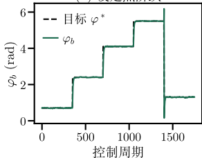
(b) 设定点阶跃
