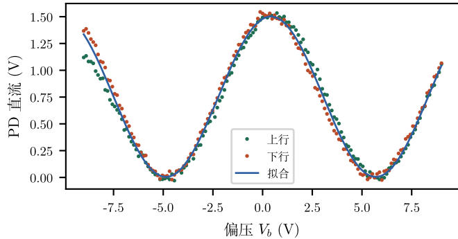
(a) 直流传递曲线 V_\pi = 5.278 V (上/下 5.358/5.197)
