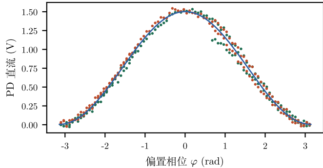
(b) 直流-相位曲线
