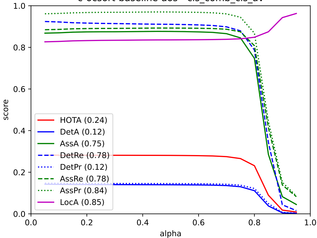
c-ocsort-baseline-aos - cls_comb_cls_av
