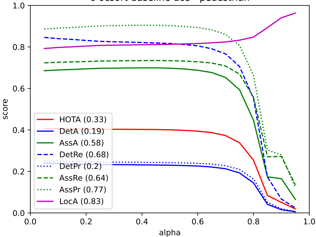
c-ocsort-baseline-aos - pedestrian
