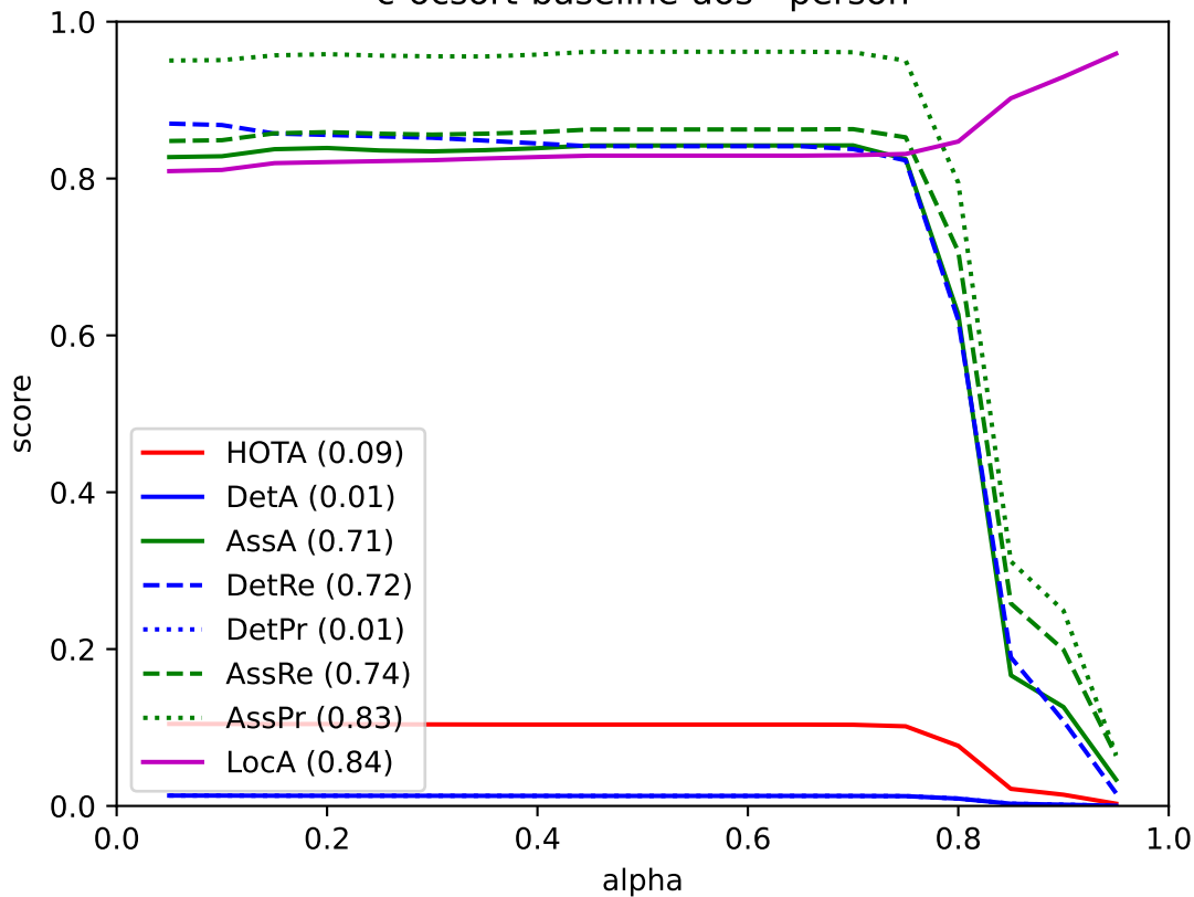
c-ocsort-baseline-aos - person
