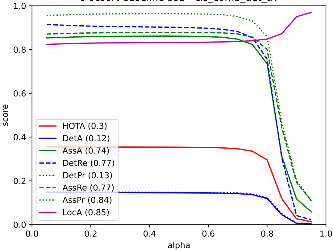
c-ocsort-baseline-soa - cls_comb_det_av
