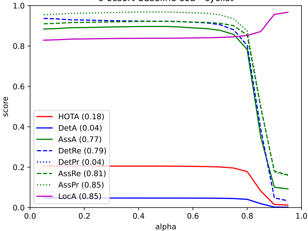
c-ocsort-baseline-soa - cyclist
