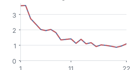
V-JEPA 2.1 [C]
