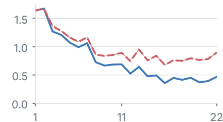
V-JEPA 2.1 [C]
