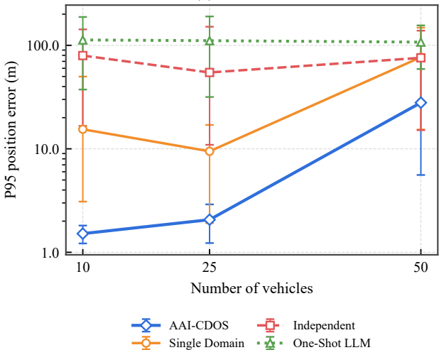
(d) Position Error
