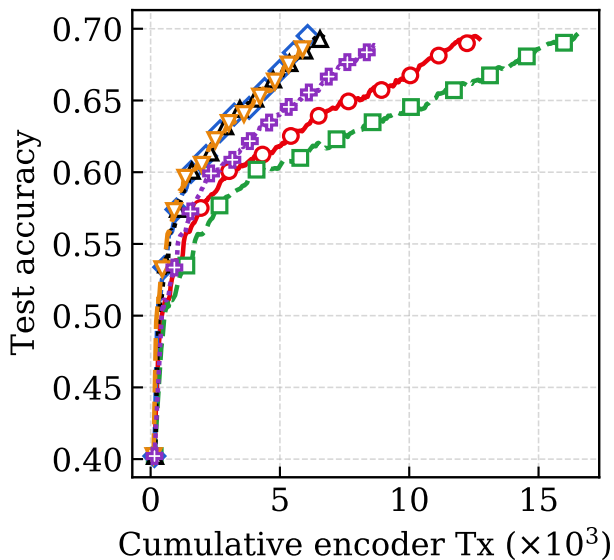
(b) nuScenes
