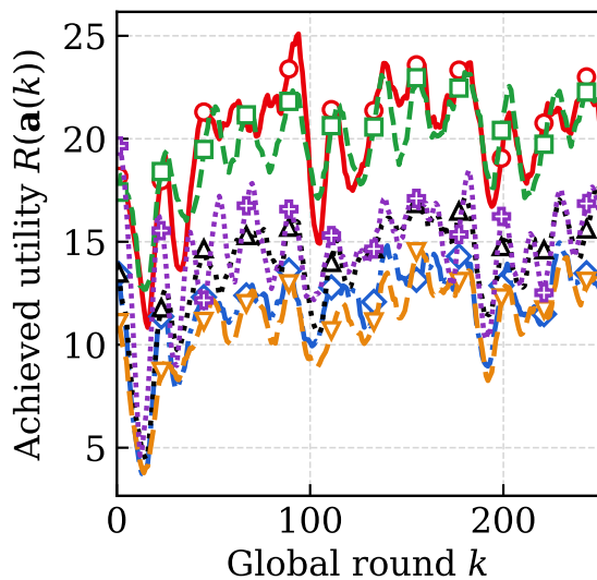
(b) nuScenes
